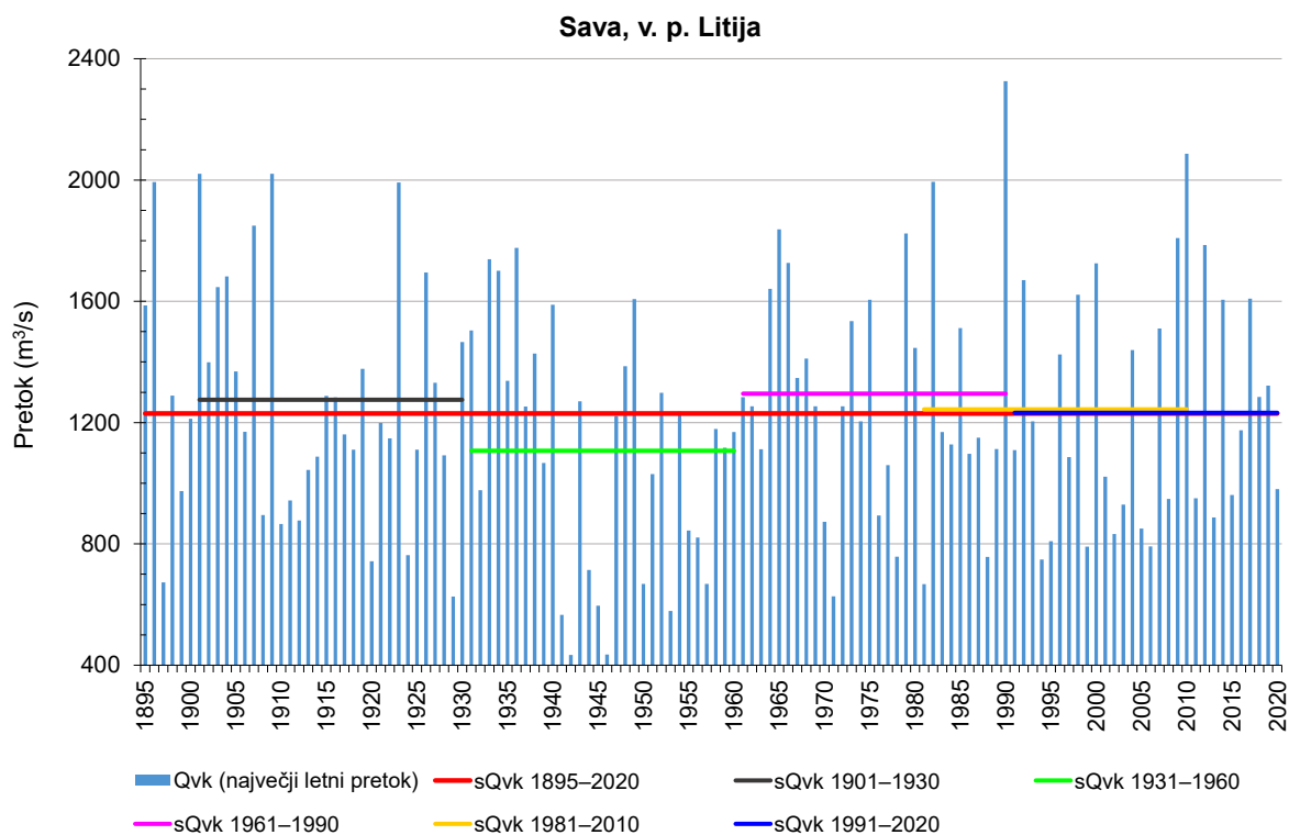
Slika 10: Letne visokovodne konice, povprečje obdobja 1895–2020 in 30-letna povprečja visokovodnih konic Save na vodometri postaji Litija
