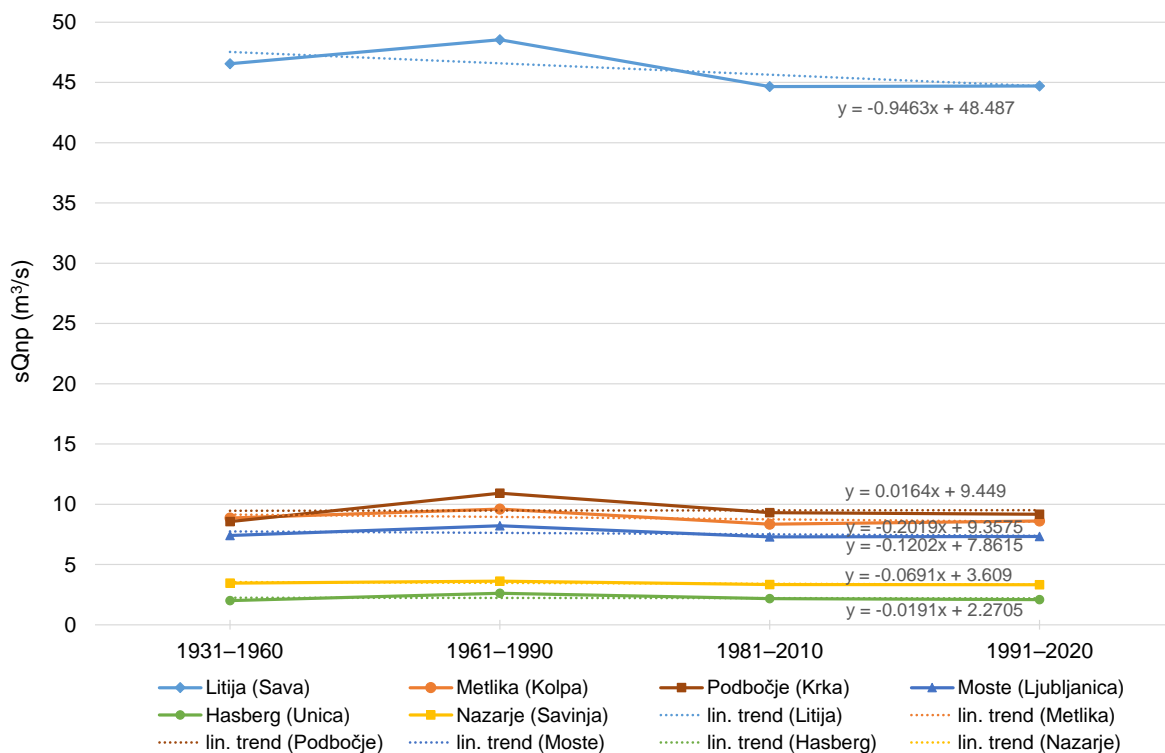
Slika 6: Srednji mali obdobjni pretoki za 30-letna obdobja 1931–1960, 1961–1990, 1981–2010 in 1991–2020 za obravnavane vodomerne postaje ter linearni trend
