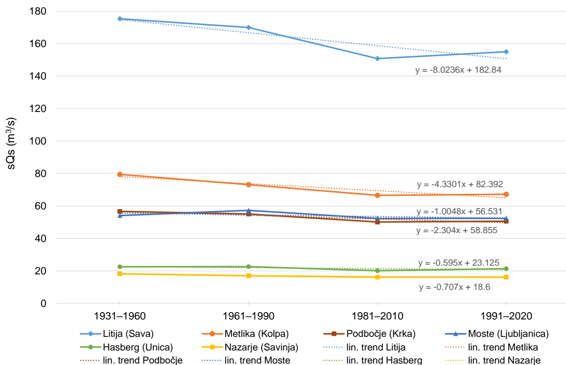
Slika 3: Srednji obdobjni pretoki za 30-letna obdobja 1931–1960, 1961–1990, 1981–2010 in 1991–2020 za obravnavane vodomerne postaje ter linearni trend
