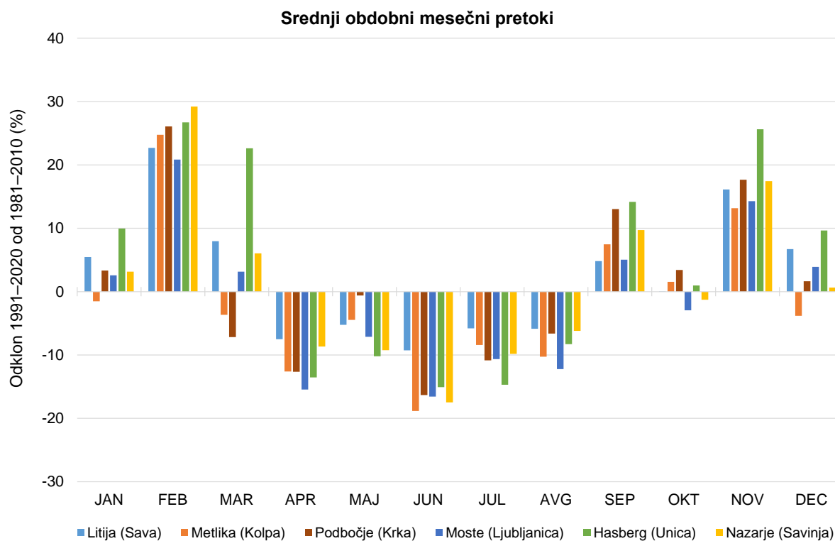
Slika 13: Odklon srednjih obdobjnih mesečnih pretokov obdobja 1991–2020 od obdobja 1981–2010 za obravnavane vodomerne postaje
