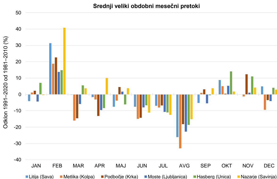
Slika 15: Odklon srednjih velikih obdobjnih mesečnih pretokov (visokovodnih konic) obdobja 1991–2020 od obdobja 1981–2010 za obravnavane vodomerne postaje
