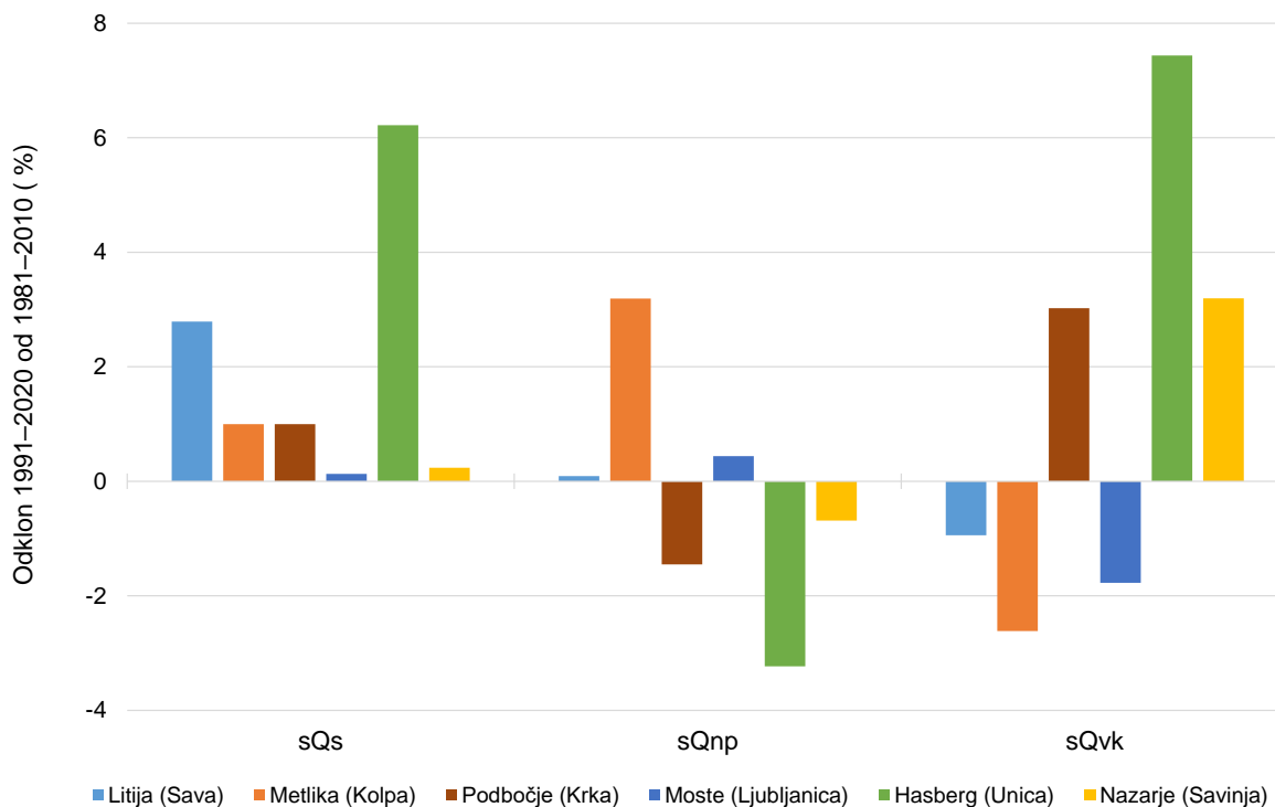
Slika 12: Odklon značilnih obdobjnih pretokov obdobja 1991–2020 od obdobja 1981–2010 za obravnavane vodomerne postaje
