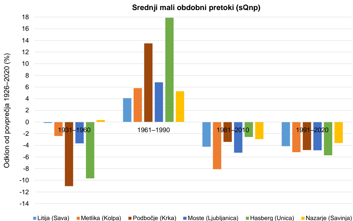
Slika 8: Odklon srednjih malih obdobjnih pretokov od povprečja obdobja 1926–2020
