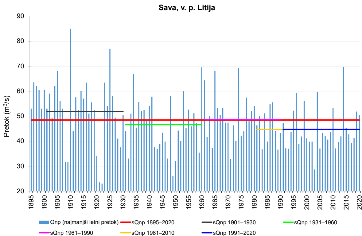
Slika 7: Najmanjši letni pretoki, povprečje obdobja 1895–2020 in 30-letna povprečja najmanjših letnih pretokov Save na vodomerni postaji Litija
