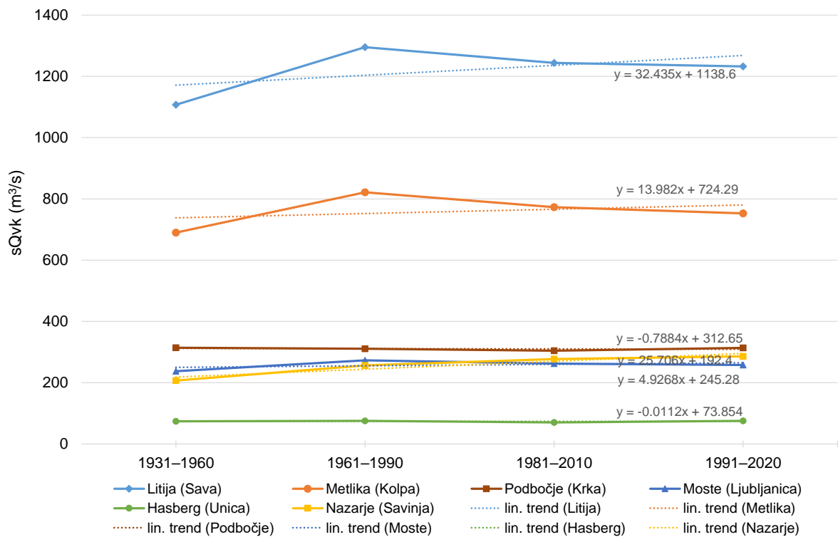
Slika 9: Srednje obdobjne visokovodne konice za 30-letna obdobja 1931–1960, 1961–1990, 1981–2010 in 1991–2020 za obravnavane vodomerne postaje ter linearni trend
