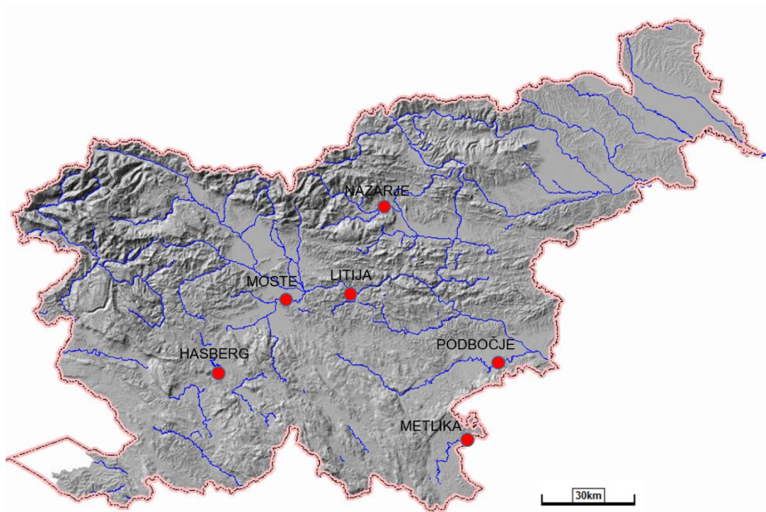
Slika 2: Lokacije obravnavanih vodomernih postaj
