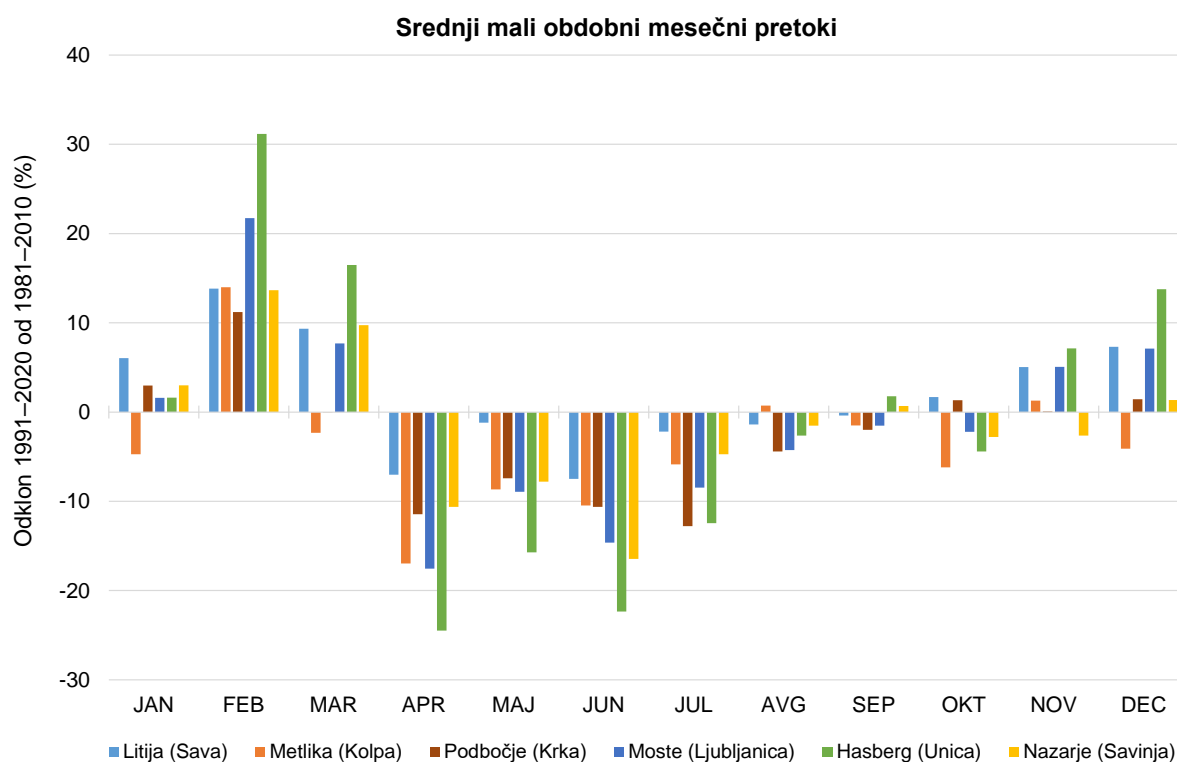
Slika 14: Odklon srednjih malih obdobjnih mesečnih pretokov obdobja 1991–2020 od obdobja 1981–2010 za obravnavane vodomerne postaje
