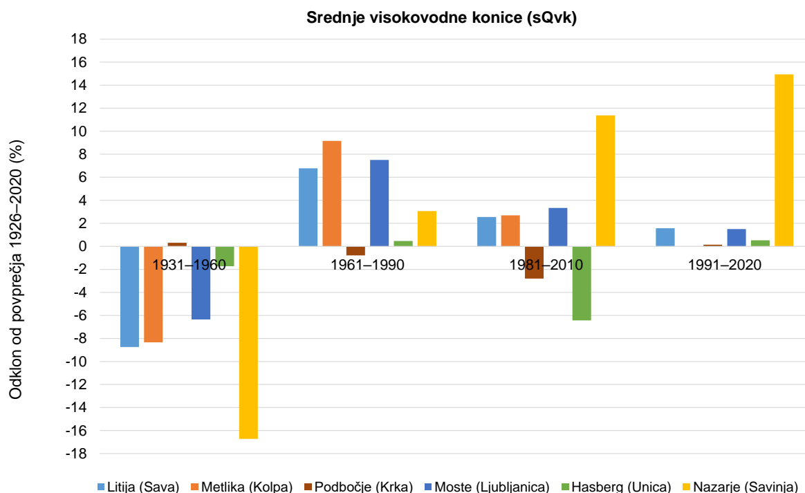
Slika 11: Odklon srednjih obdobjnih visokovodnih konic od povprečja obdobja 1926–2020
