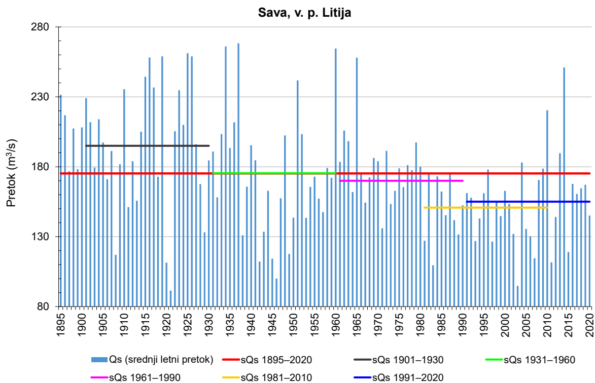
Slika 4: Srednji letni pretoki, povprečje obdobja 1895–2020 in 30-letna povprečja srednjih pretokov Save na vodomerni postaji Litija
